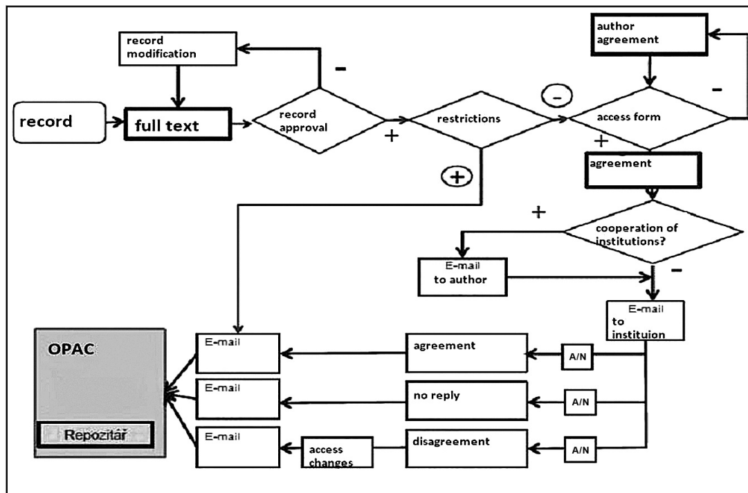
Obr. 3 Workflow institucionálního repozitáře
